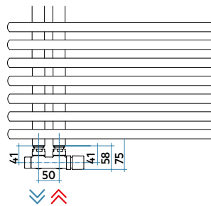
Instalare cu colectori în stânga Conexiune hidraulică 50 mm
